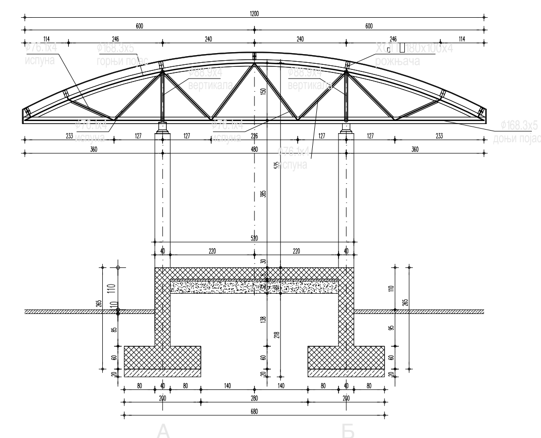
ПОПРЕЧНИ ПРЕСЕК 4-4
