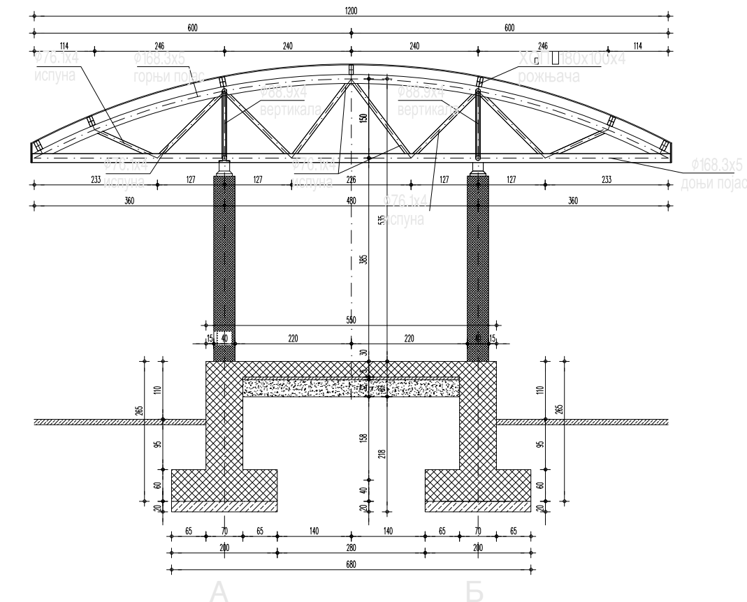
ПОПРЕЧНИ ПРЕСЕК 3-3
