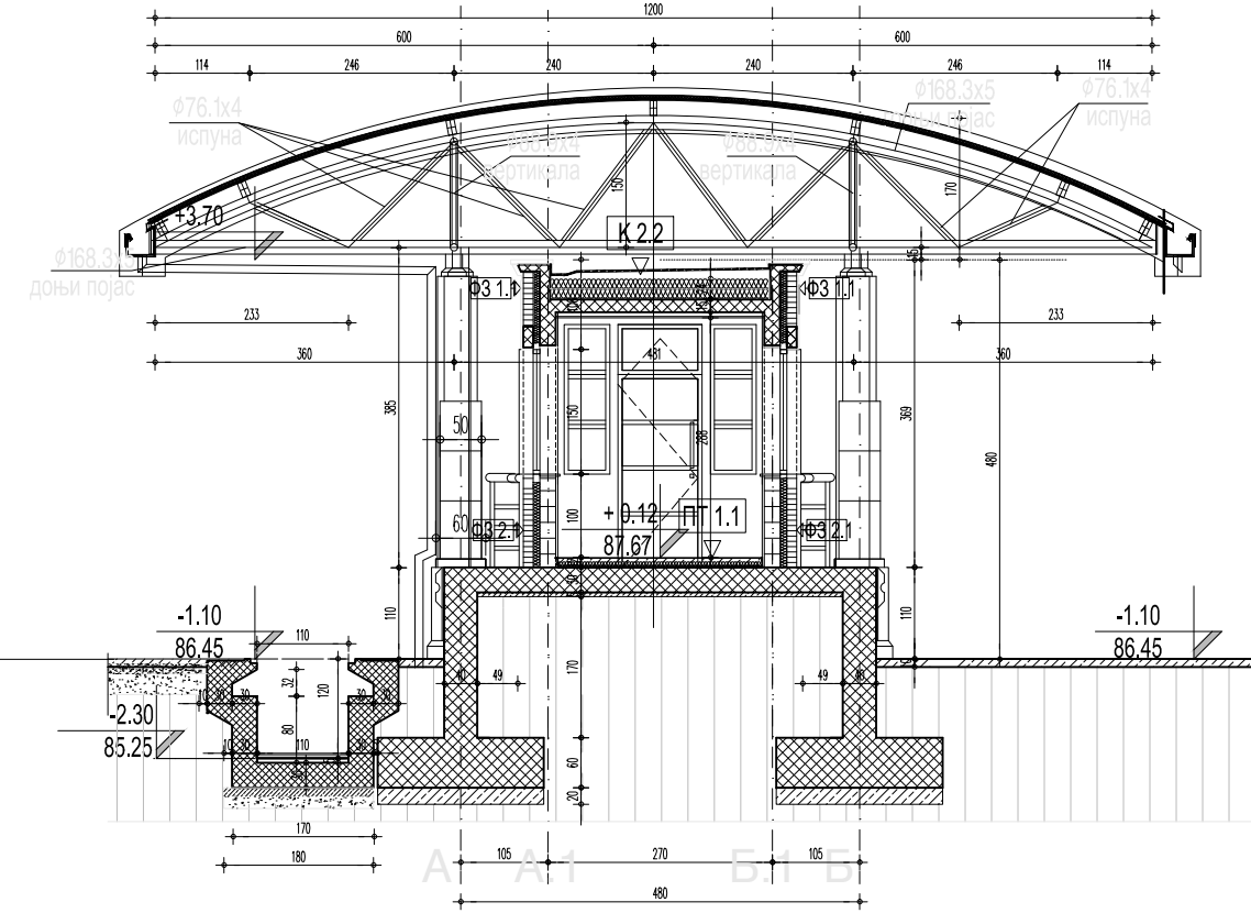
ПОПРЕЧНИ ПРЕСЕК 1
