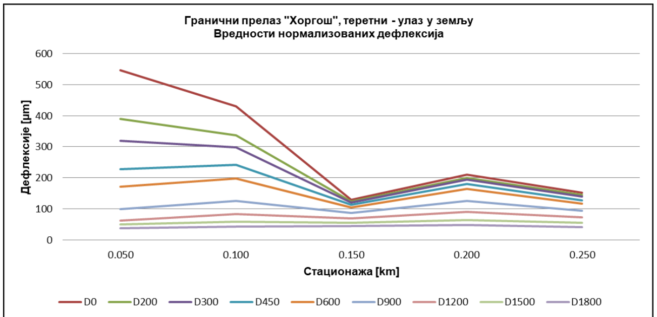
Слика 4.2.1.5 Дијаграм вредности нормализованих дефлексија, ГП „Хоргош“ – теретни терминал улаз у земљу (прве 2 тачке на асфалтном коловозу, следеће 3 тачке на бетонском коловозу)
