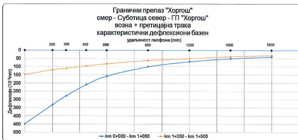
Слика 12 – карактеристични дефлексиони базен – смер Суботица север – ГП „Хоргош“
