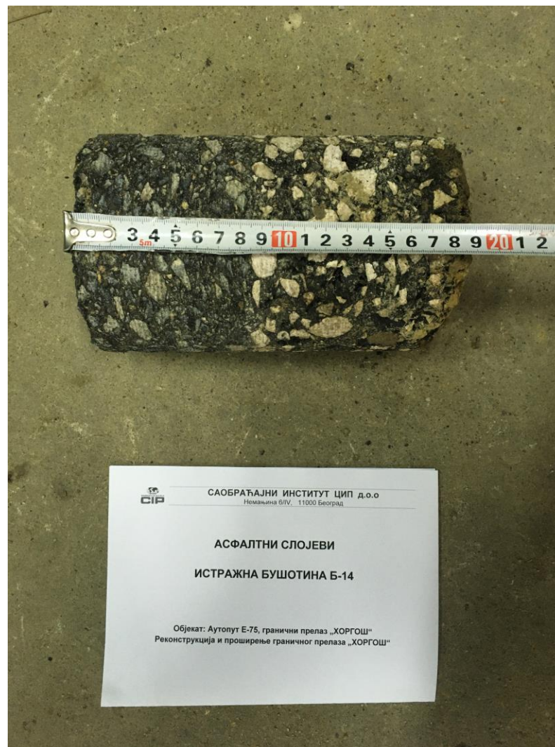
Слика П16.12 Узорак асфалтних слојева из бушотине Б – 14, km 0+073.52
