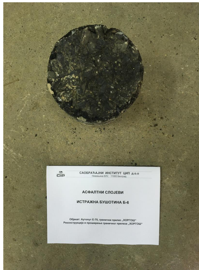
Слика П16.8 Горња површина узорка асфалтних слојева из бушотине Б – 6, km 0+423.02
