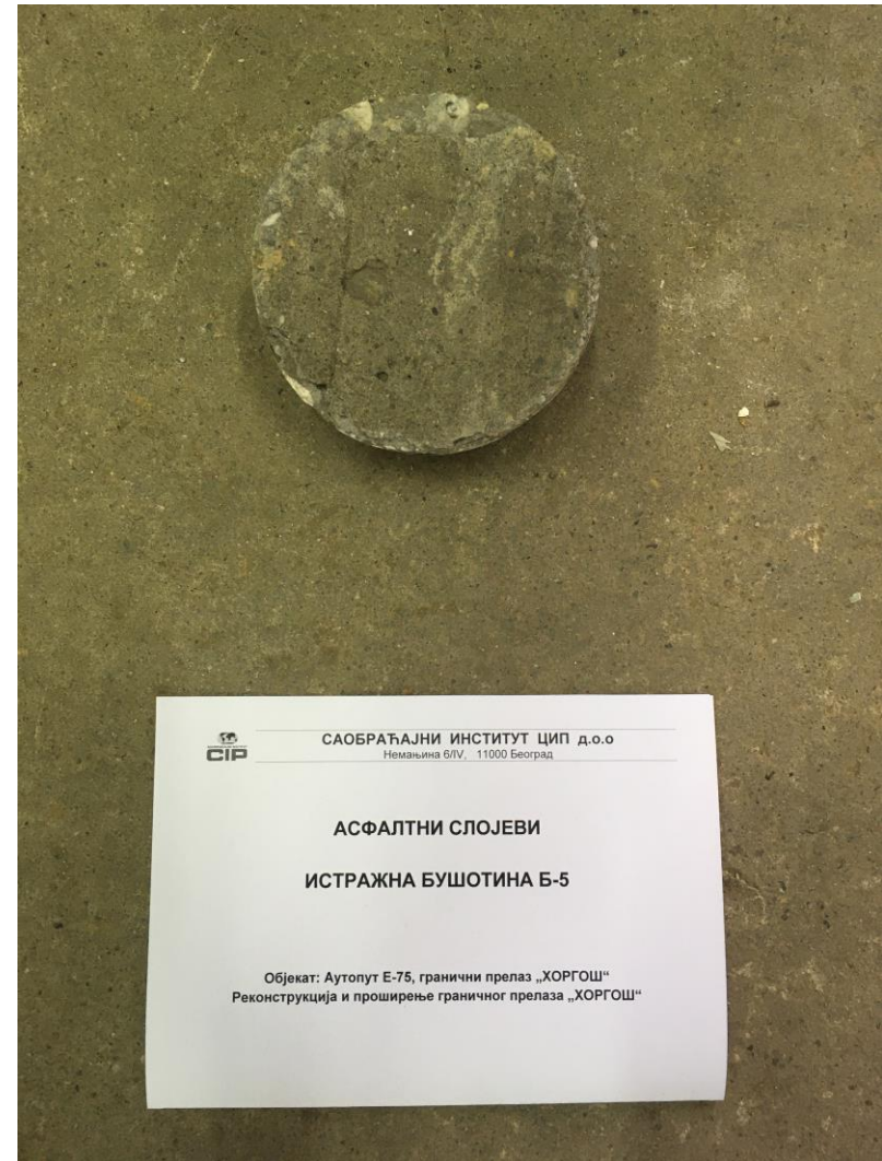
Слика П16.6 Горња површина узорка бетонског застора из бушотине Б – 5, km 0+497.93
