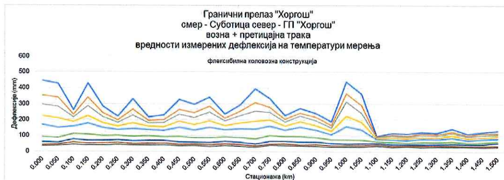
Слика 4 – дијаграм вредности измерених дефлексија на температури мерења, смер Суботица север – ГП „Хоргош“ – возна + претицајна трака
