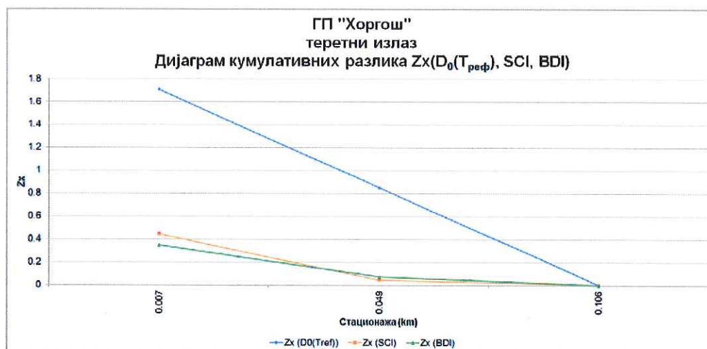
Слика 10 – дијаграм кумулативних разлика Z_x(D_0(T_{\text{реф}})) , Z_x(BDI) и Z_x(SCI) ГП „Хоргош“ – Теретни излаз
