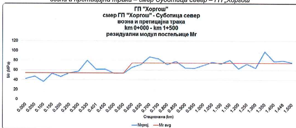
Слика 26 – резидуални модул постелџице возна и претицајна трака – смер ГП „Хоргош“ – Суботица север
