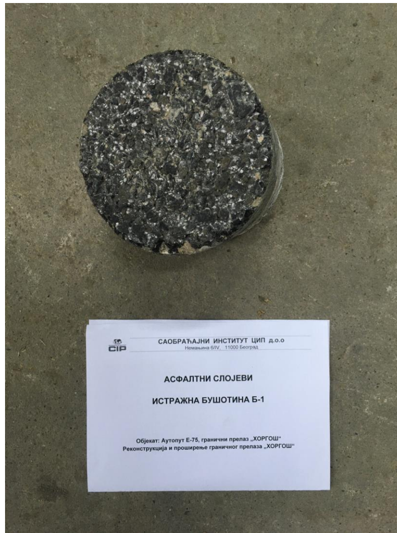
Слика П16.2 Горња површина узорка асфалтних слојева из бушотине Б – 1, km 1+258,38
