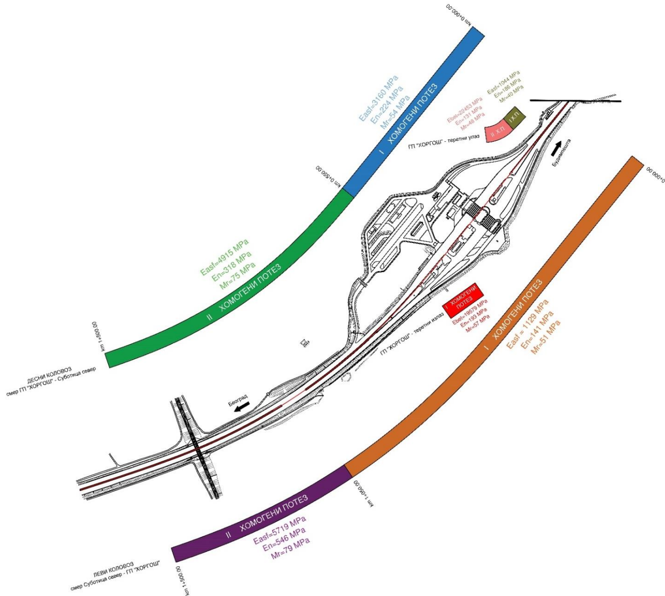
Слика 4.2.3.5. Шематски приказ хомогених потеза по тракама на ГП „Хоргош“ 2019 – 620 – 10 – САО – K2/3
