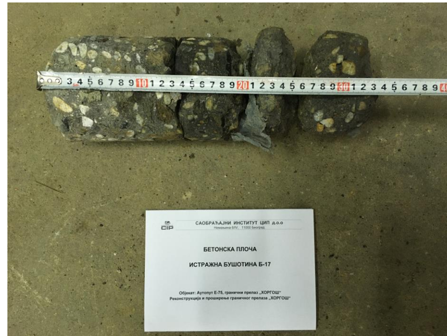
Слика П16.16 Узорак бетонског застора из бушотине Б – 17, km 0+366.40
