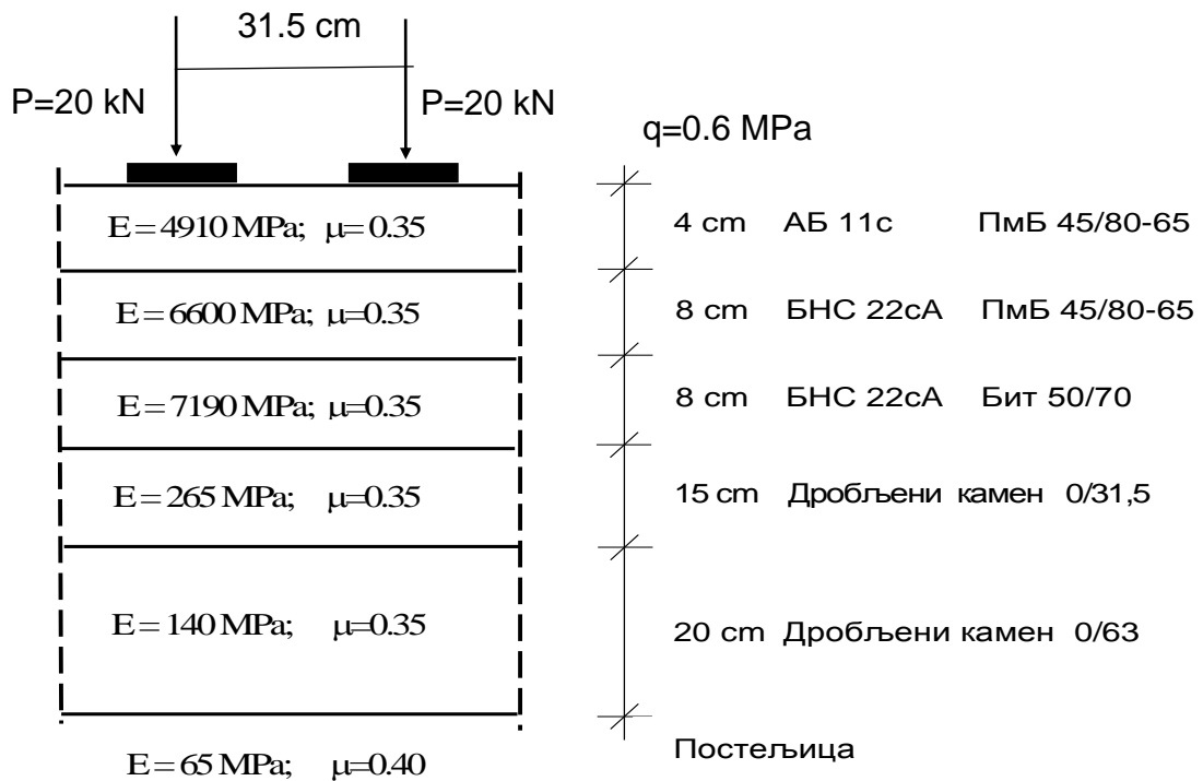
Слика 7.1.2. Прорачунски модел коловозне конструкције
