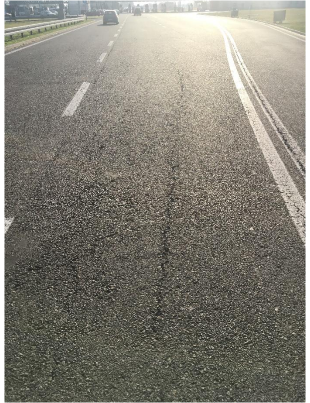
Слика 4.1.25. Подужна пукотина са разгранатом мрежом малих пукотина
