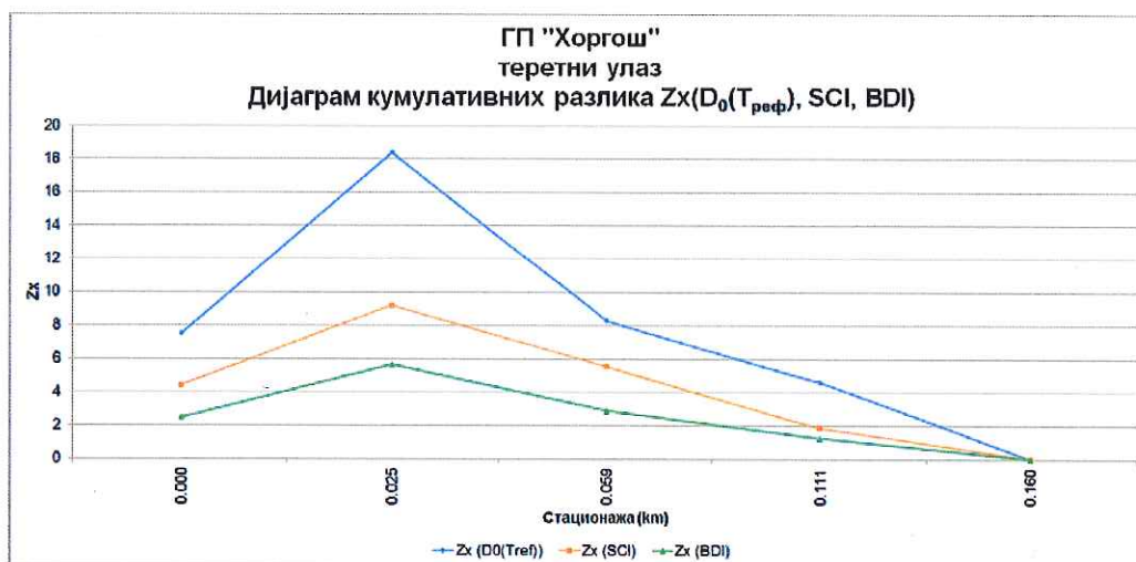
Слика 11 – дијаграм кумулативних разлика Z_x(D_0(T_{\text{реф}})) , Z_x(BDI) и Z_x(SCI) ГП „Хоргош“ – Теретни улаз
