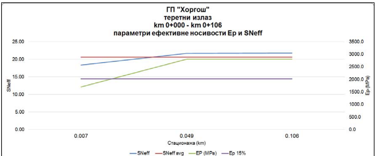
Слика 4.2.4.3 Параметри ефективне носивости, ГП „Хоргош“ – теретни излаз из земље
