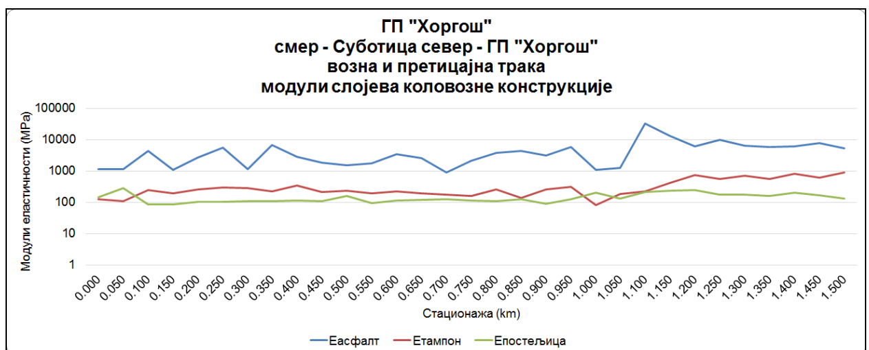
Слика 4.2.3.1 Модули еластичности слојева коловозне конструкције, смер Суботица север – ГП „Хоргош“
