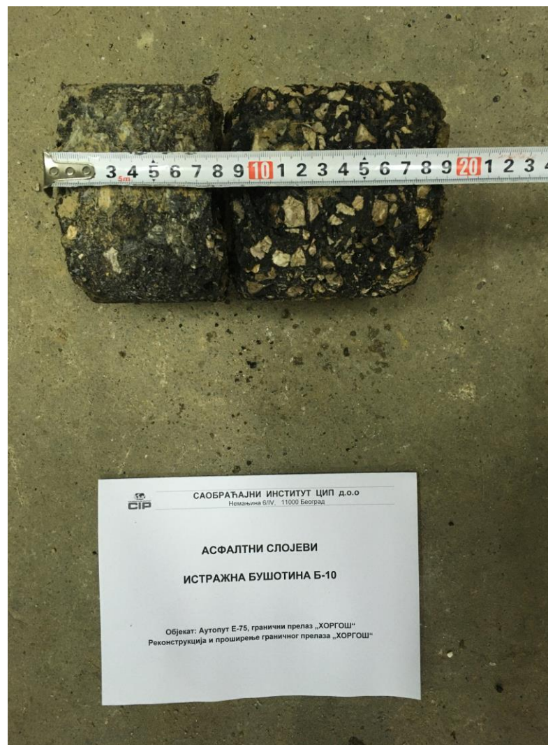
Слика П16.10 Узорак асфалтних слојева из бушотине Б – 10, km 0+296.49
